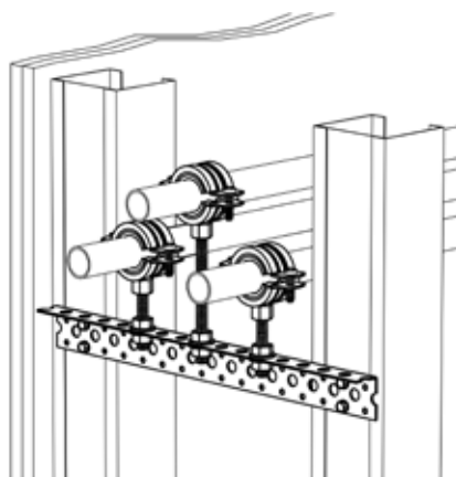
Montagevoorbeeld voor horizontale leidingen
