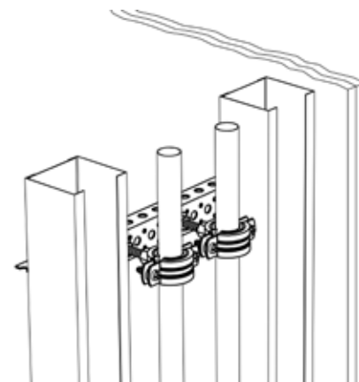
Montagevoorbeeld voor verticale leidingen
